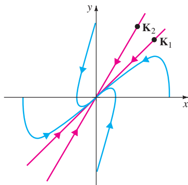
FIGURA 10.2.3 Nodo estable.
